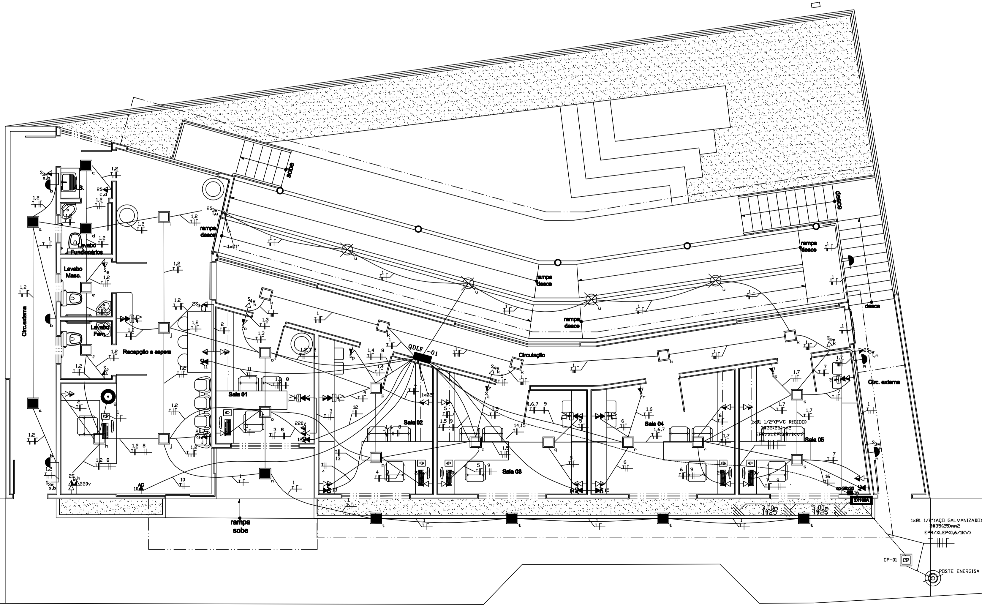
PLANTA BAIXA TÉRREO (ILUMINAÇÃO E TOMADAS) ESCALA 1 : 50
