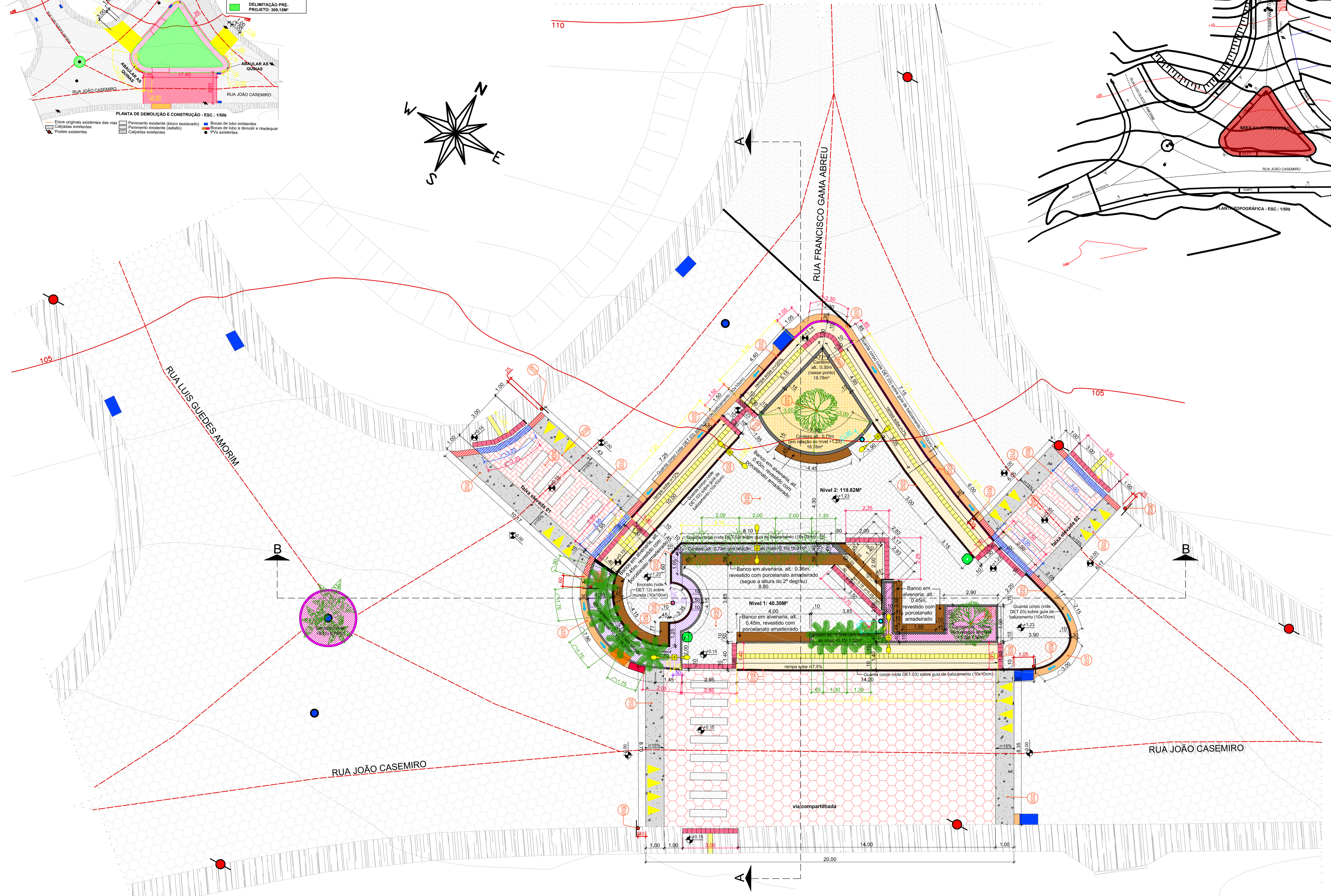
Planta Baixa Escala: 1/100
