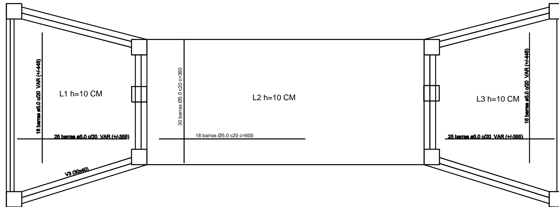
ARMAÇÃO POSITIVA DAS LAJES DA FUNDAÇÃO (X, Y) ESCALA 1:50
